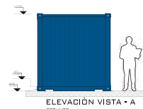
ELEVACIÓN VISTA - A ESD: 1/50
